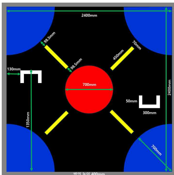
그림 3. 씨름 로봇 대회 경기장
