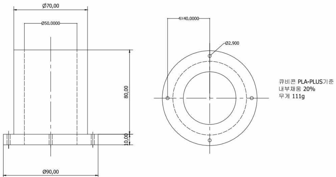
그림 2. 색깔 통 규격
